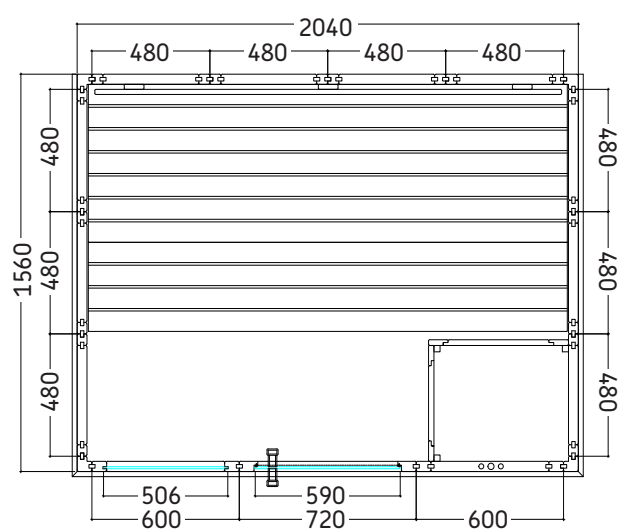
Aufbau rechts
