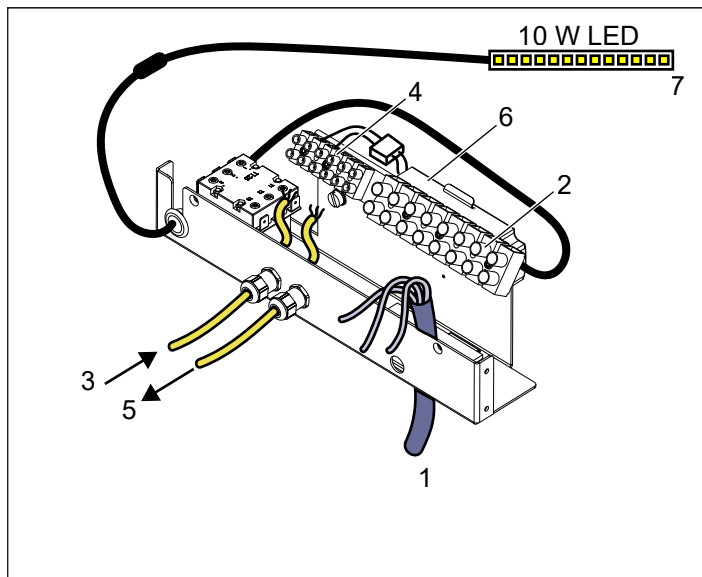
Illustration 9: Compartiment électrique
