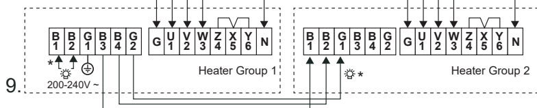
Rysunek 16F. Schemat okablowania 200–240 V ~
