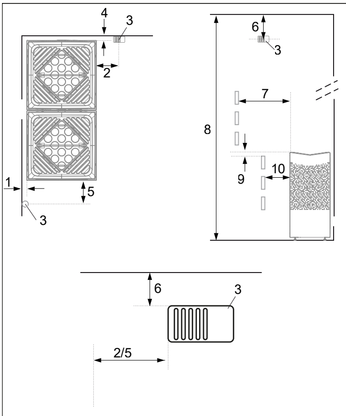
Illustration 3B : Positionnement du poêle : deux poêles de sauna
