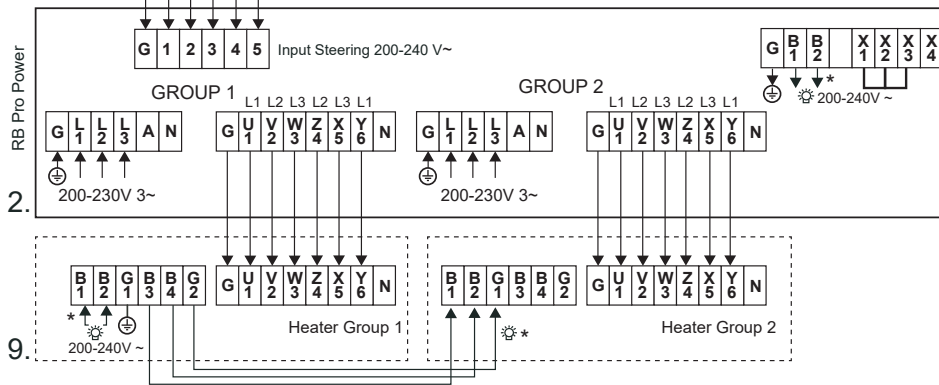
Illustration 16E : Schéma de raccordement 200-230 V 3~
