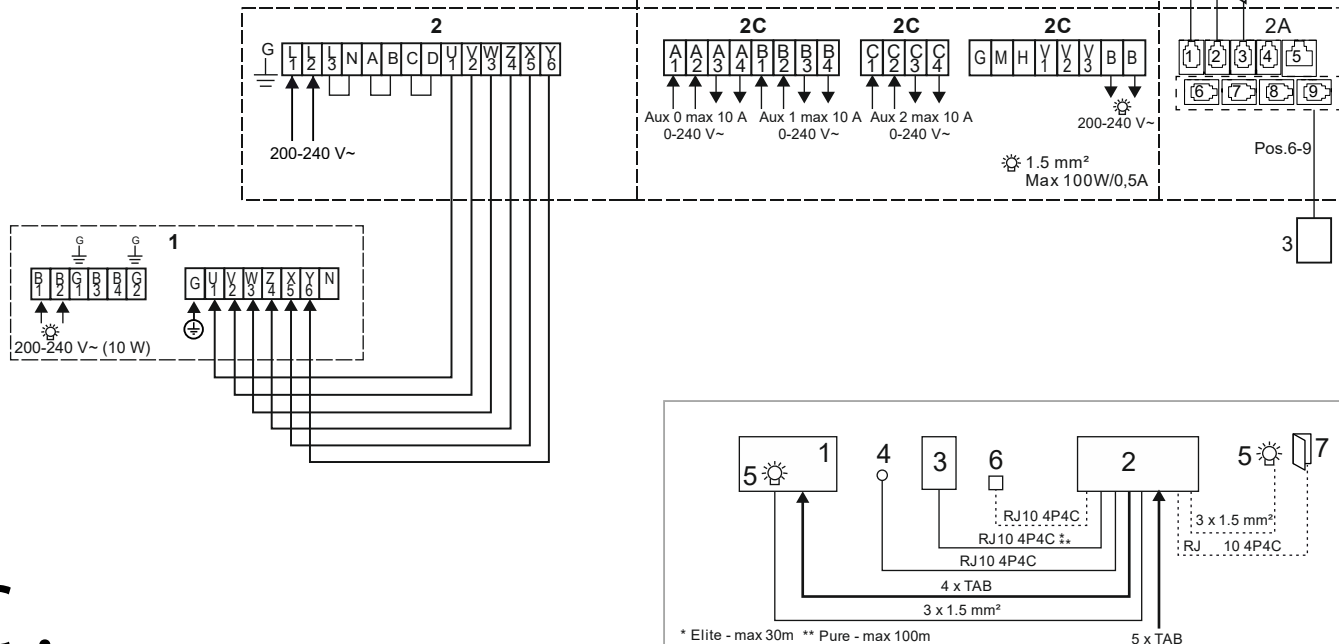
Abbildung 16C: Schaltplan 200-240 V ~
