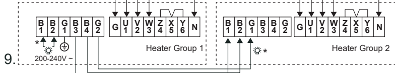
Afbeelding 16F: Bedradingsschema 230-240 V~
