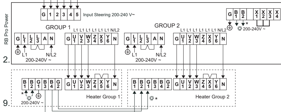
Fig 16F: Kopplingsschema, 200-240V ~
