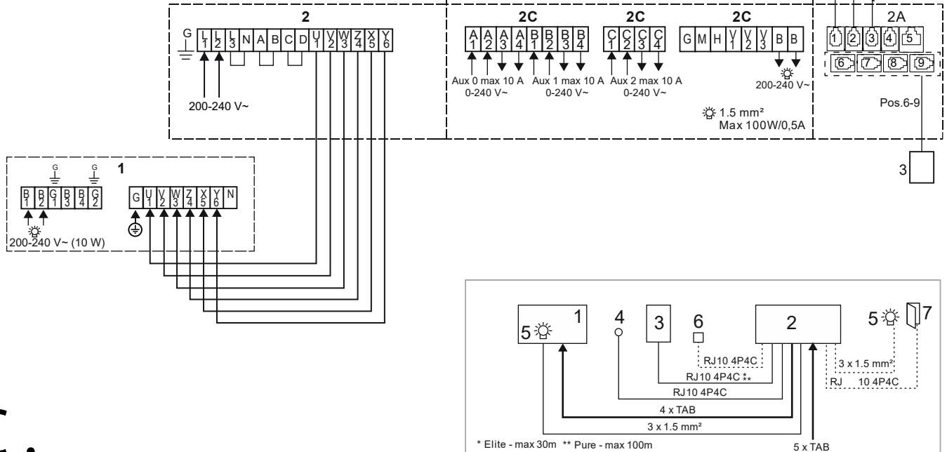
Afbeelding 16C: Bedradingsschema 230-240 V~
