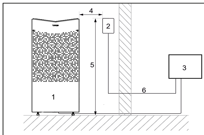
Abbildung 5: Sicherheitsabstand/Montagehöhe, Bedienpanel
