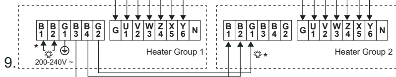
Fig 16E: Kopplingsschema, 200-230V 3~
