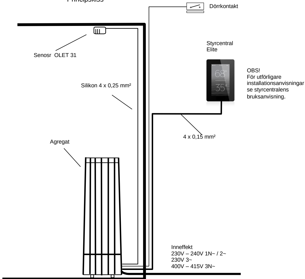
Bild 10 Principskiss
