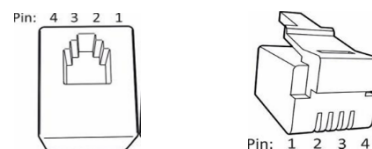
Joonis 8 Konnektori RJ10 kontaktide paigutus
