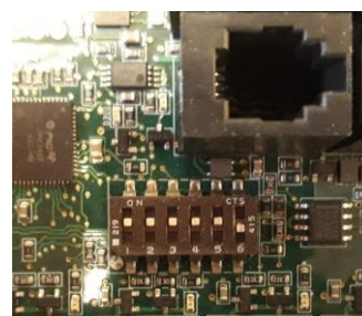
Rysunek 6 Pozycje przełączników Dip do używania grzejnika
