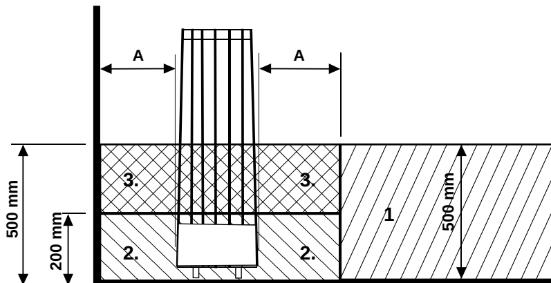
Afbeelding 5 Plaatsing van de aansluitdoos
