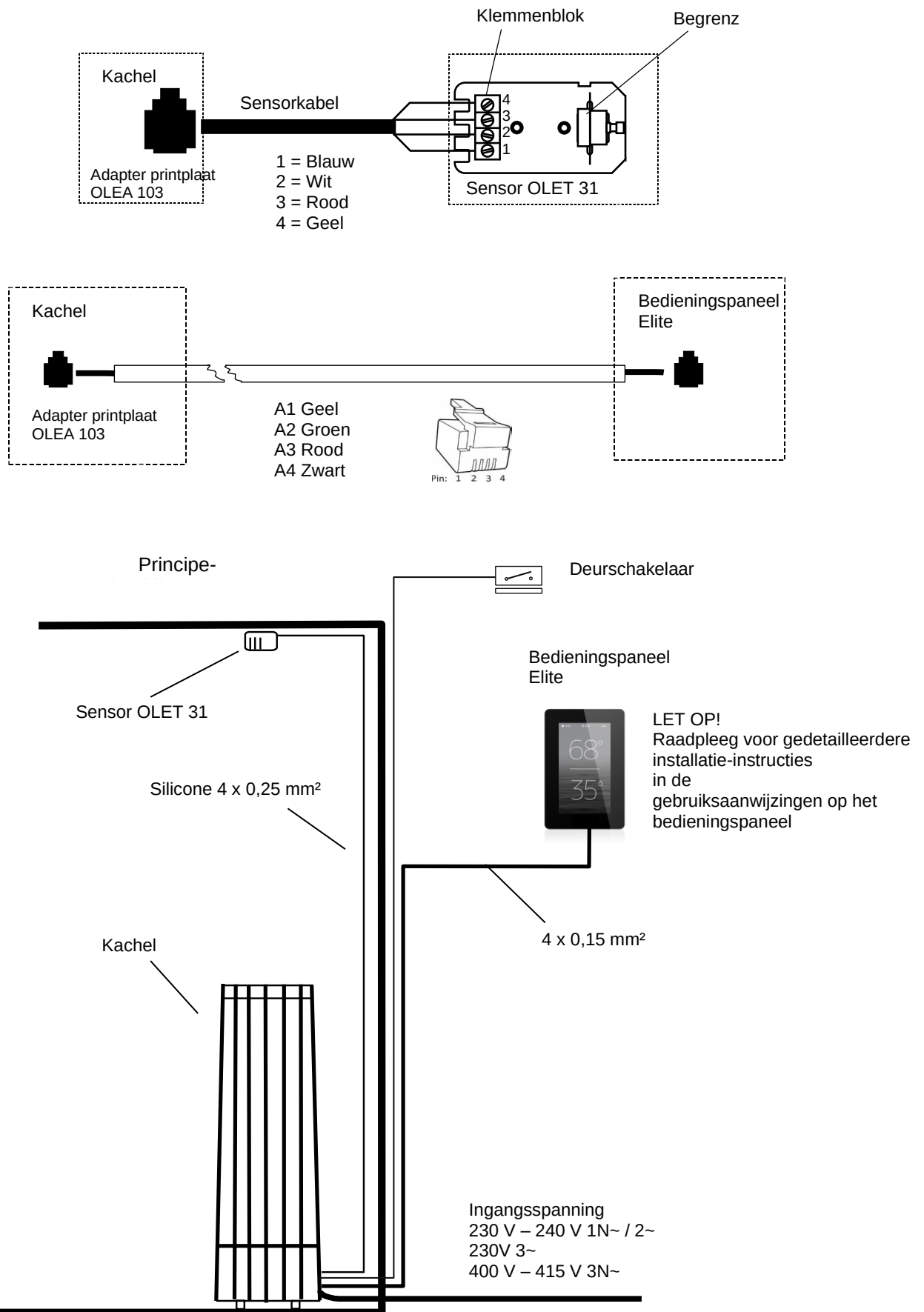
Afbeelding 10 Principe-afbeelding
