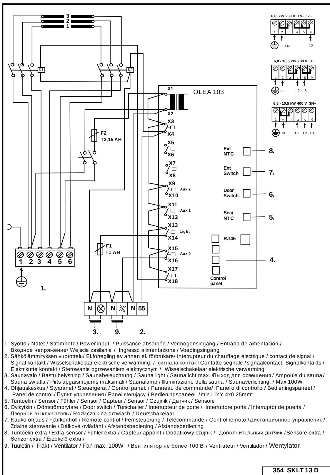
Afbeelding 9 Bedradingsschema voor de saunakachel
