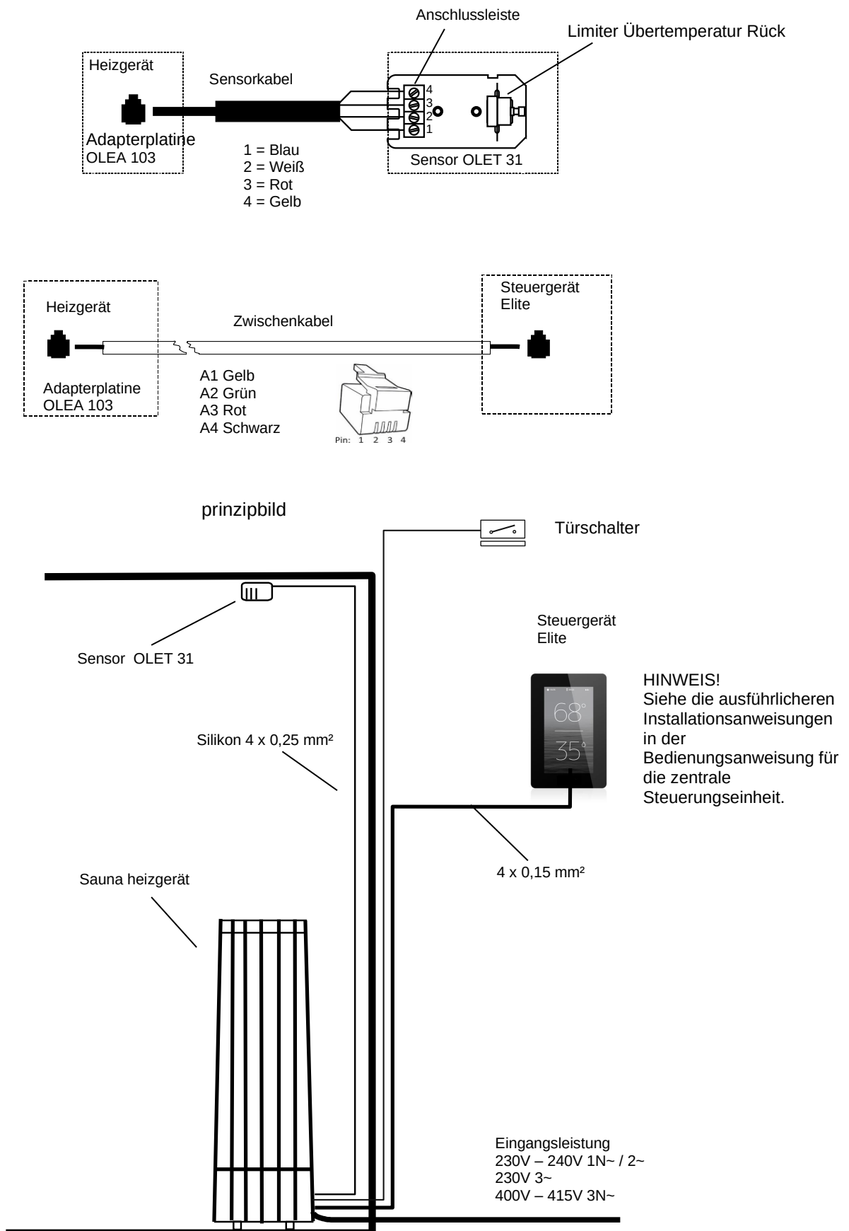
Abbildung 10 Prinzipbild
