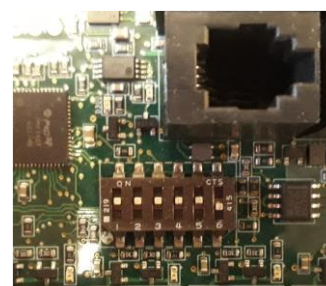
Imagen 6 Posiciones del interruptor DIP para usar un calentador
