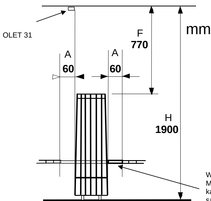
Afbeelding 2 Veiligheidsafstanden
