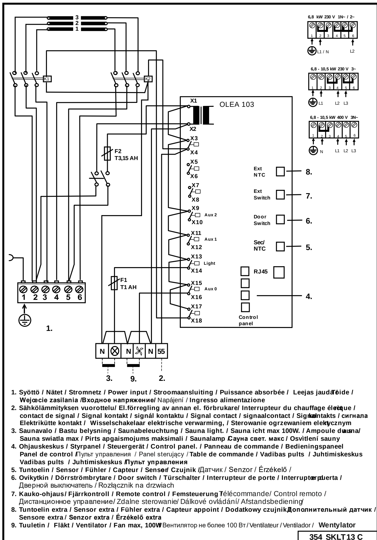
Bild 9 Kopplingsschema
