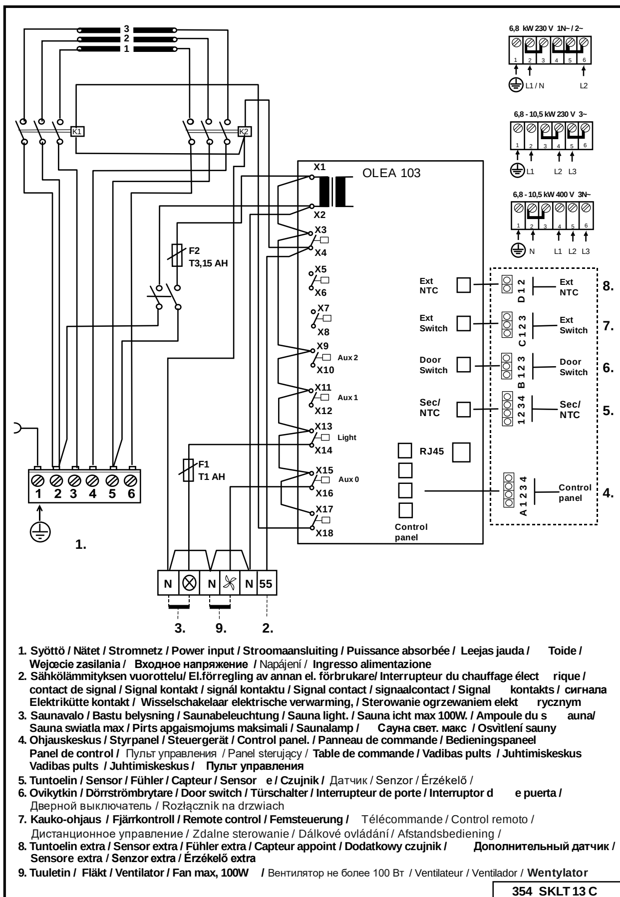
Rysunek 9 Schemat podłączenia pieca
