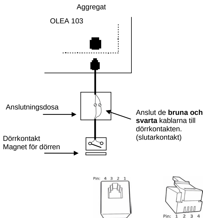
Bild 8 Stift-order av RJ 10
