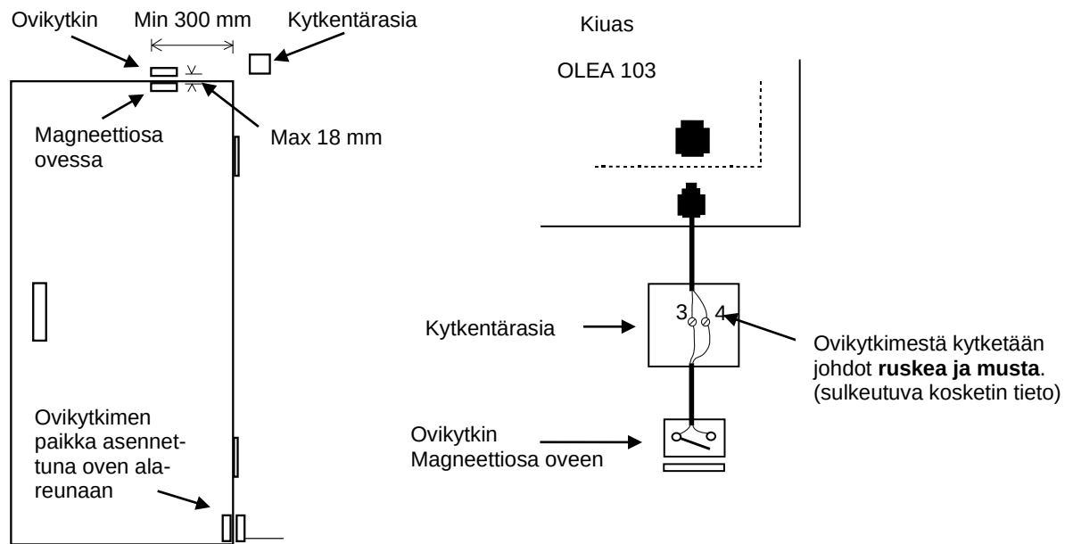
Kuva 7 Ovikytkimen asento
