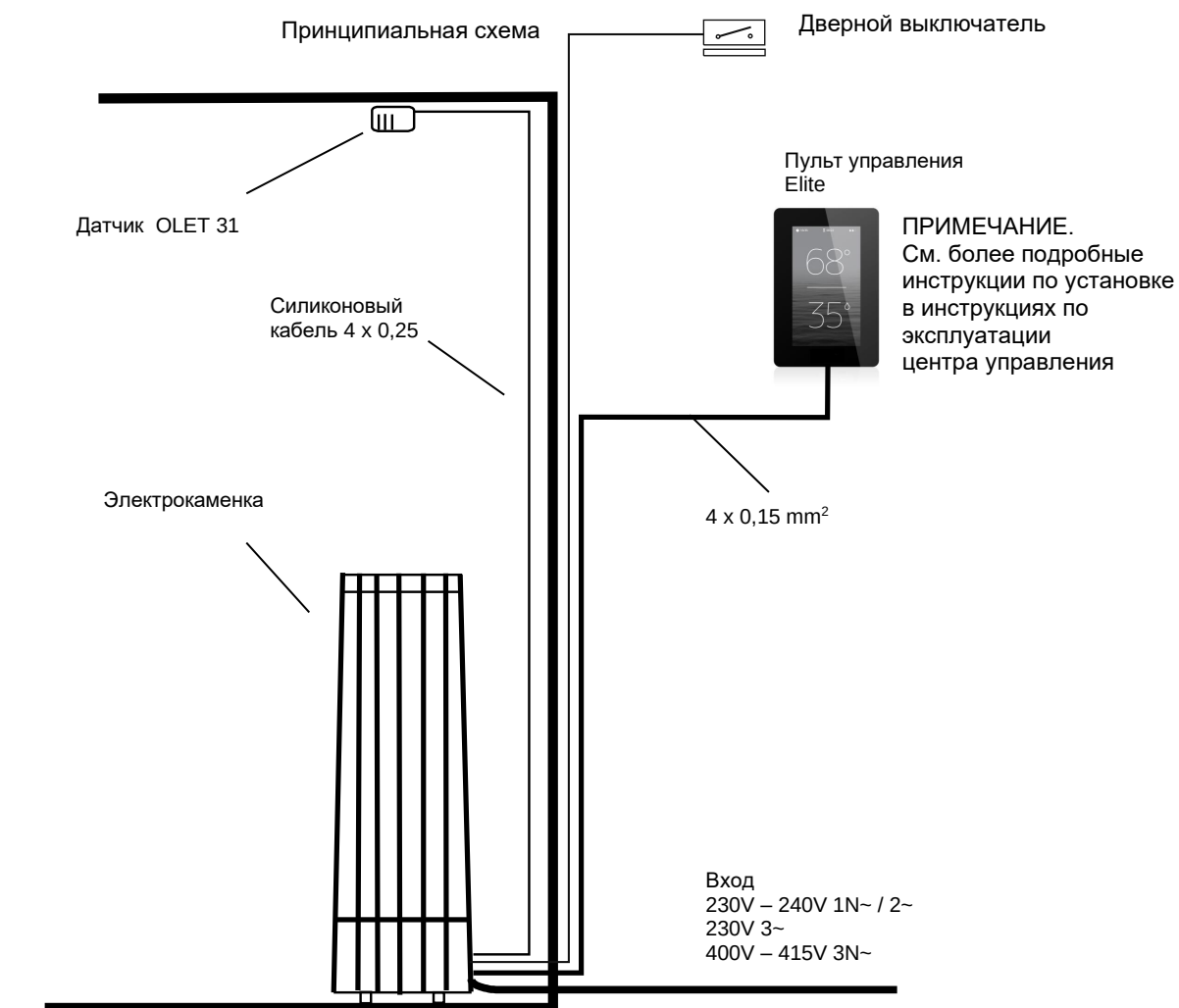
Рис 10 Принципиальная схема
