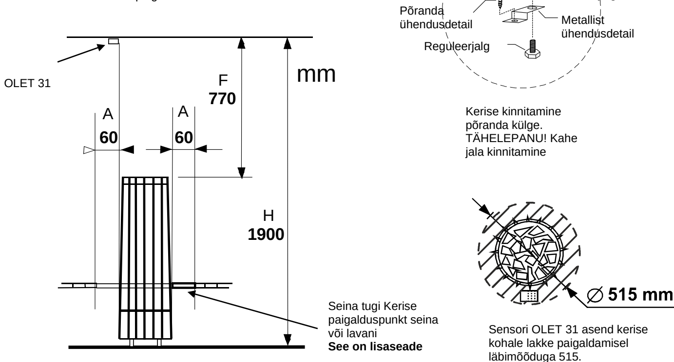
Joonis 2 Ohutusvahemikud
