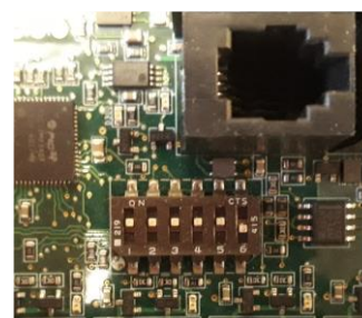
Abbildung 6 DIP-Schalterstellungen für den Betrieb eines Saunaheizgerät.
