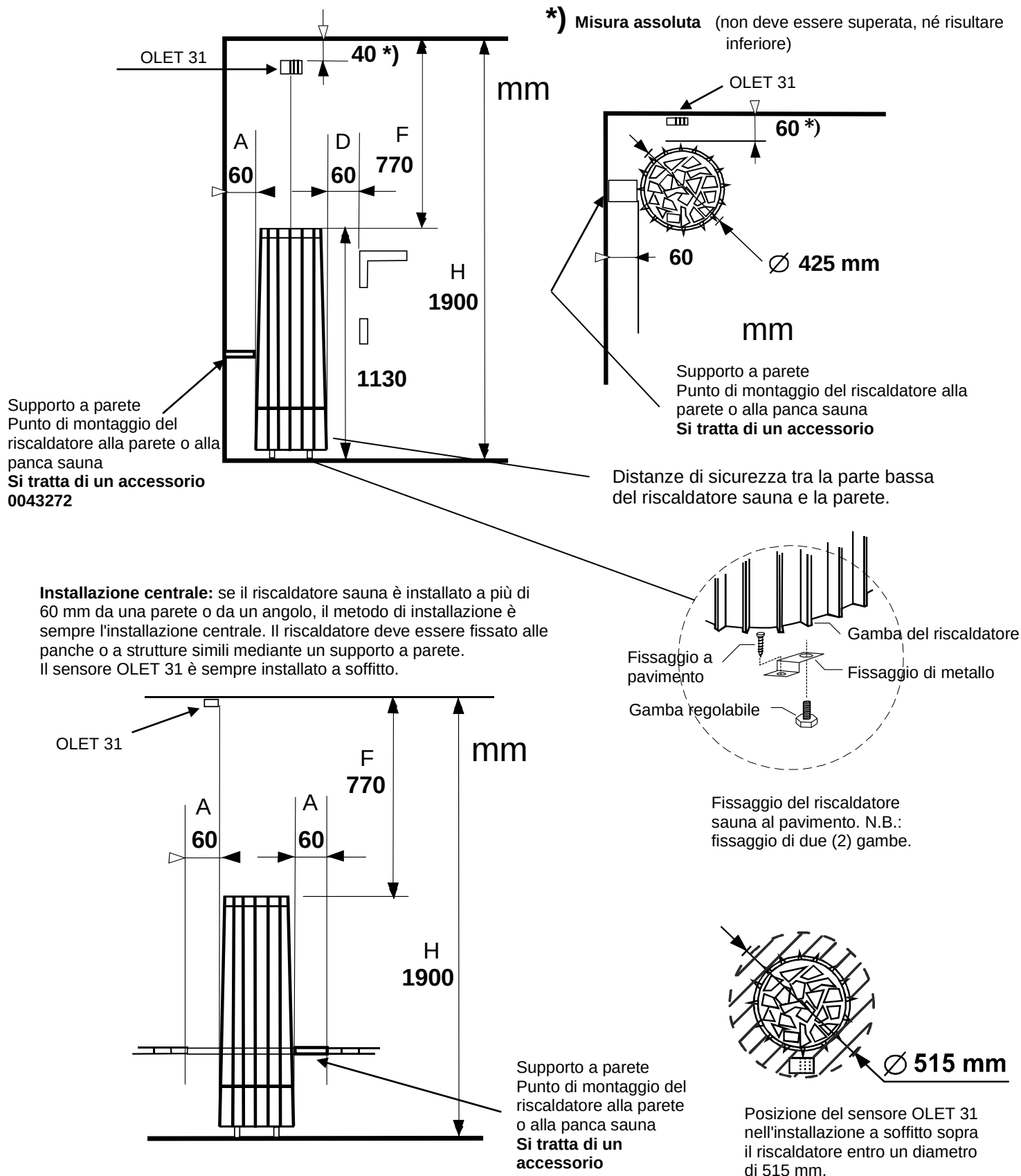
Immagine 2 Distanze di sicurezza del riscaldatore sauna
