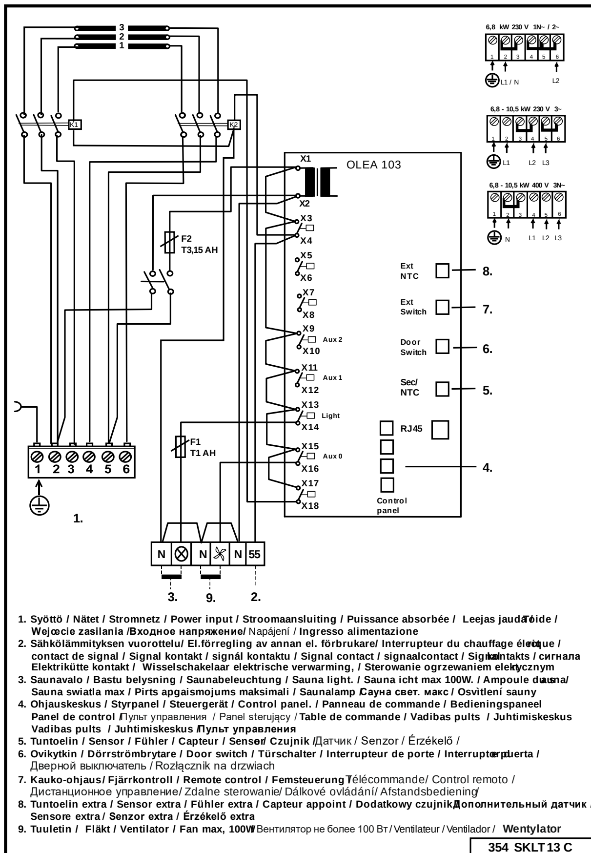
Abbildung 9 Schaltdiagramm
