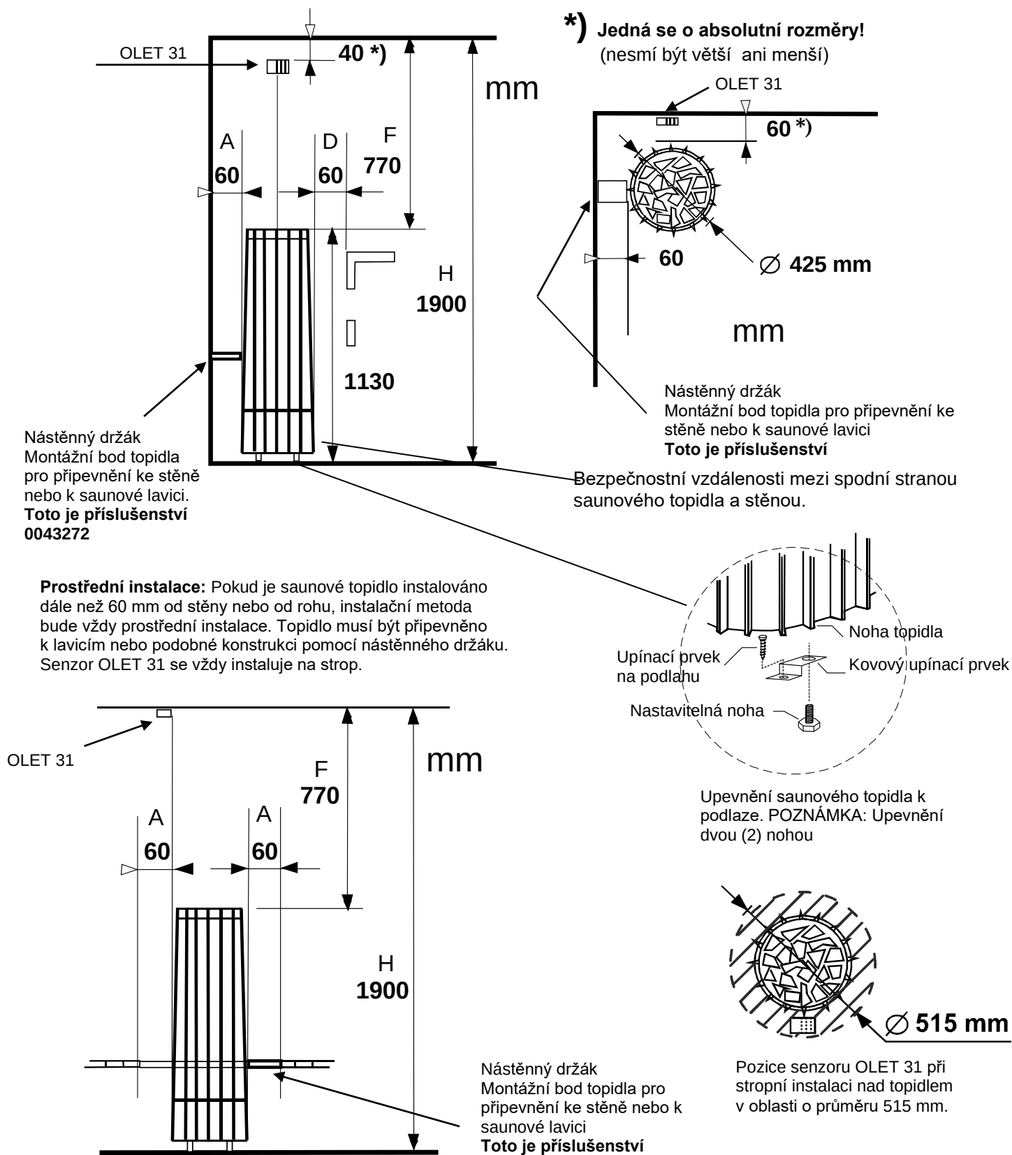
Obrázek 2 Bezpečnostní vzdálenosti saunového topidla
