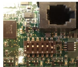
Obrázek 6 Poloha přepínačů DIP pro použití ohříváče
