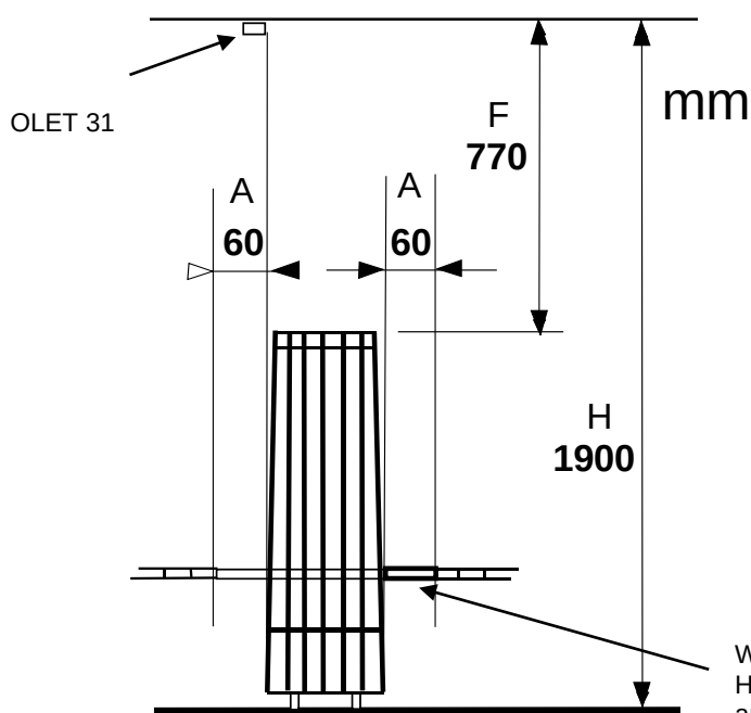
Abbildung 2 Sicherheitsabstände
