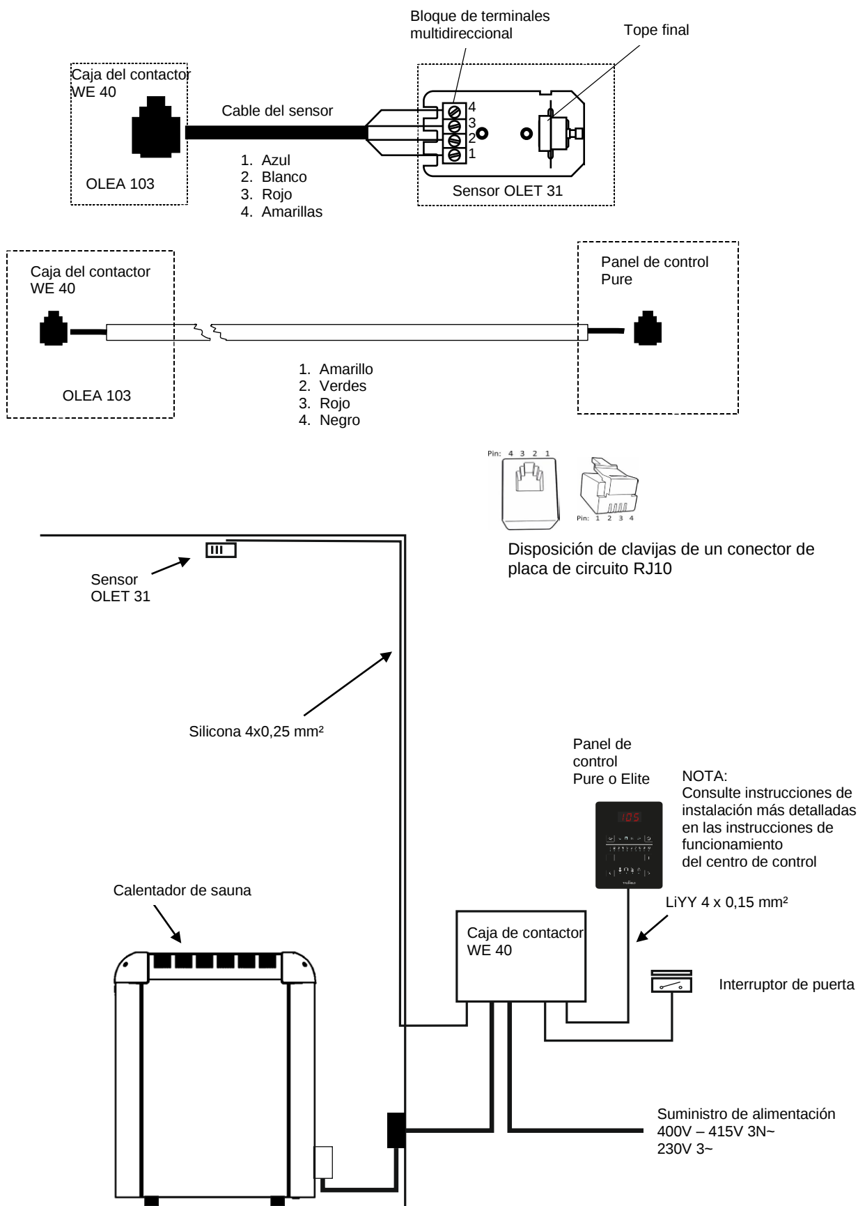
Figura 5 Diagrama del principio de conexiones
