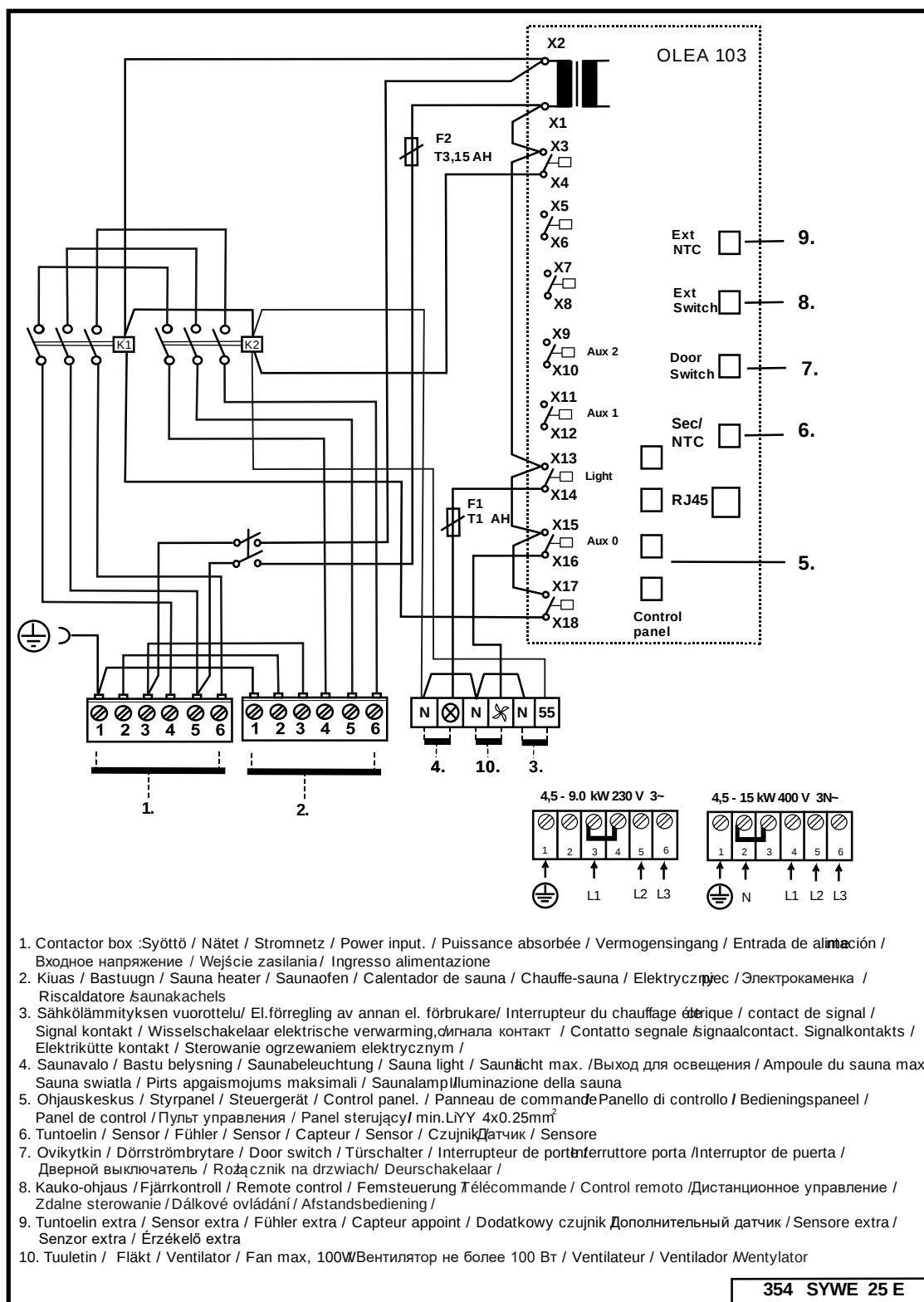
Figure 4 Schéma de raccordement box contacteur WE 40
