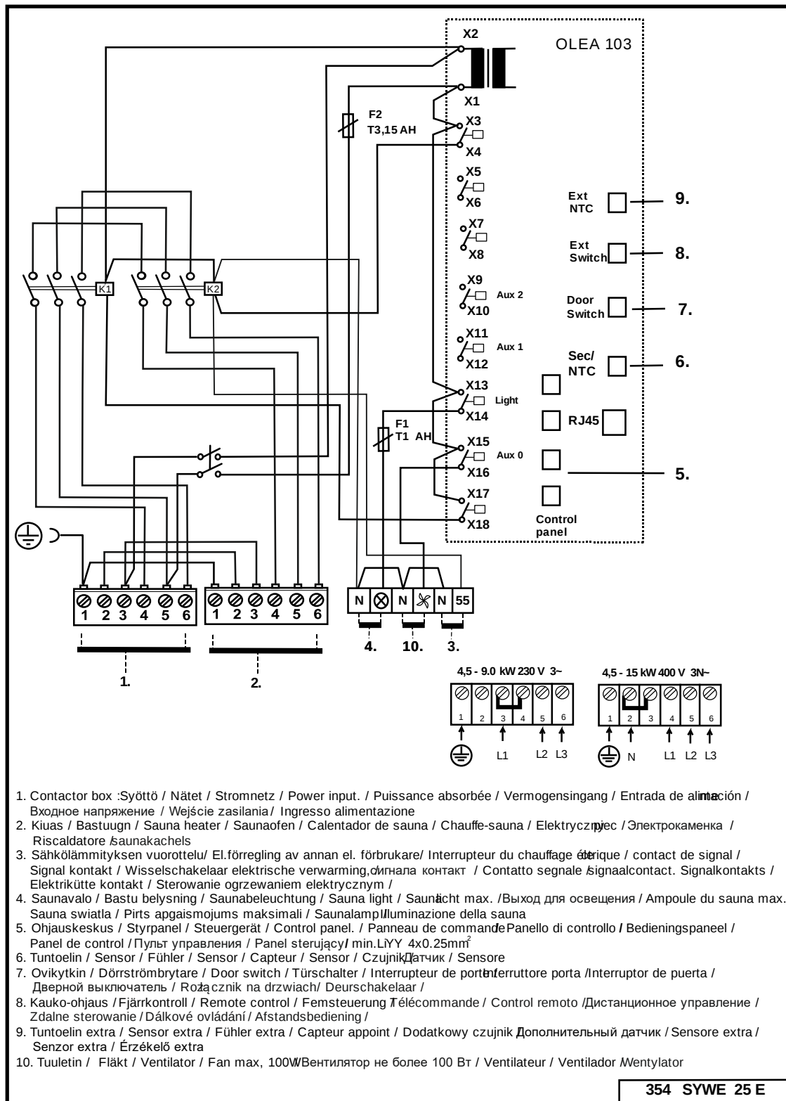
Afbeelding 4 Bedradingsschema voor de contactgever-doos WE - 40
