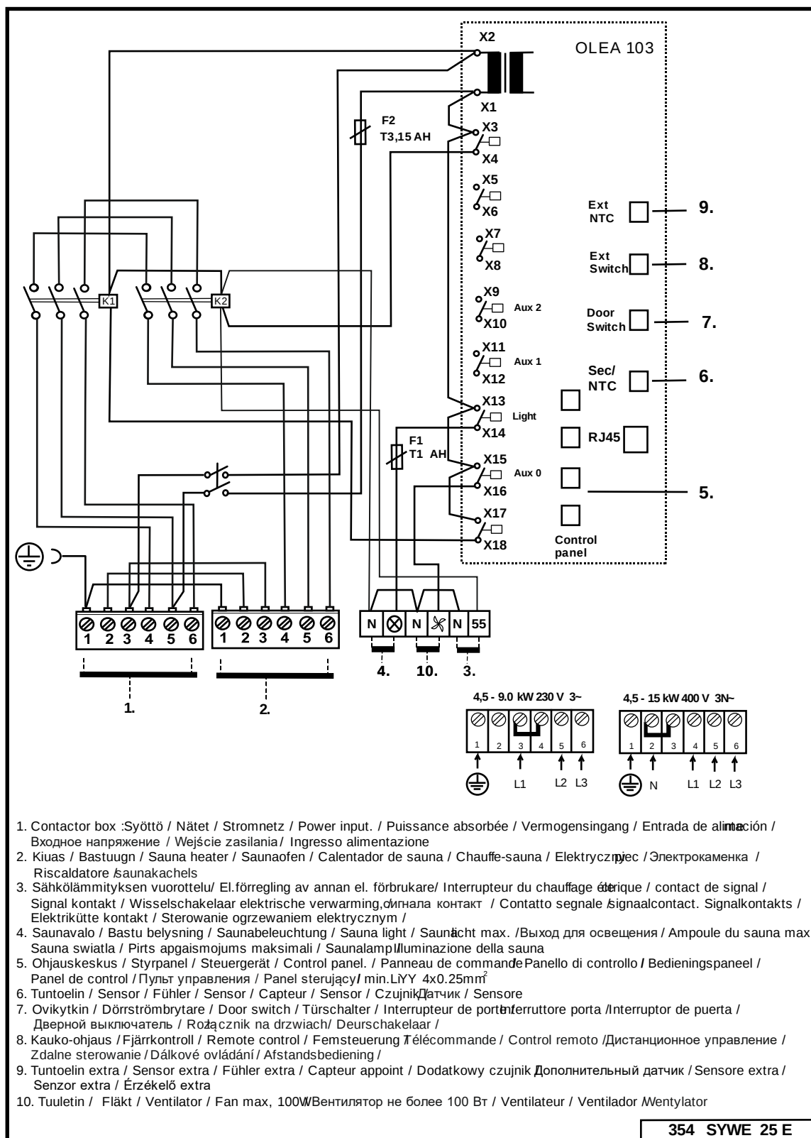
Рис. 4 Схема электрических соединений WE 40
