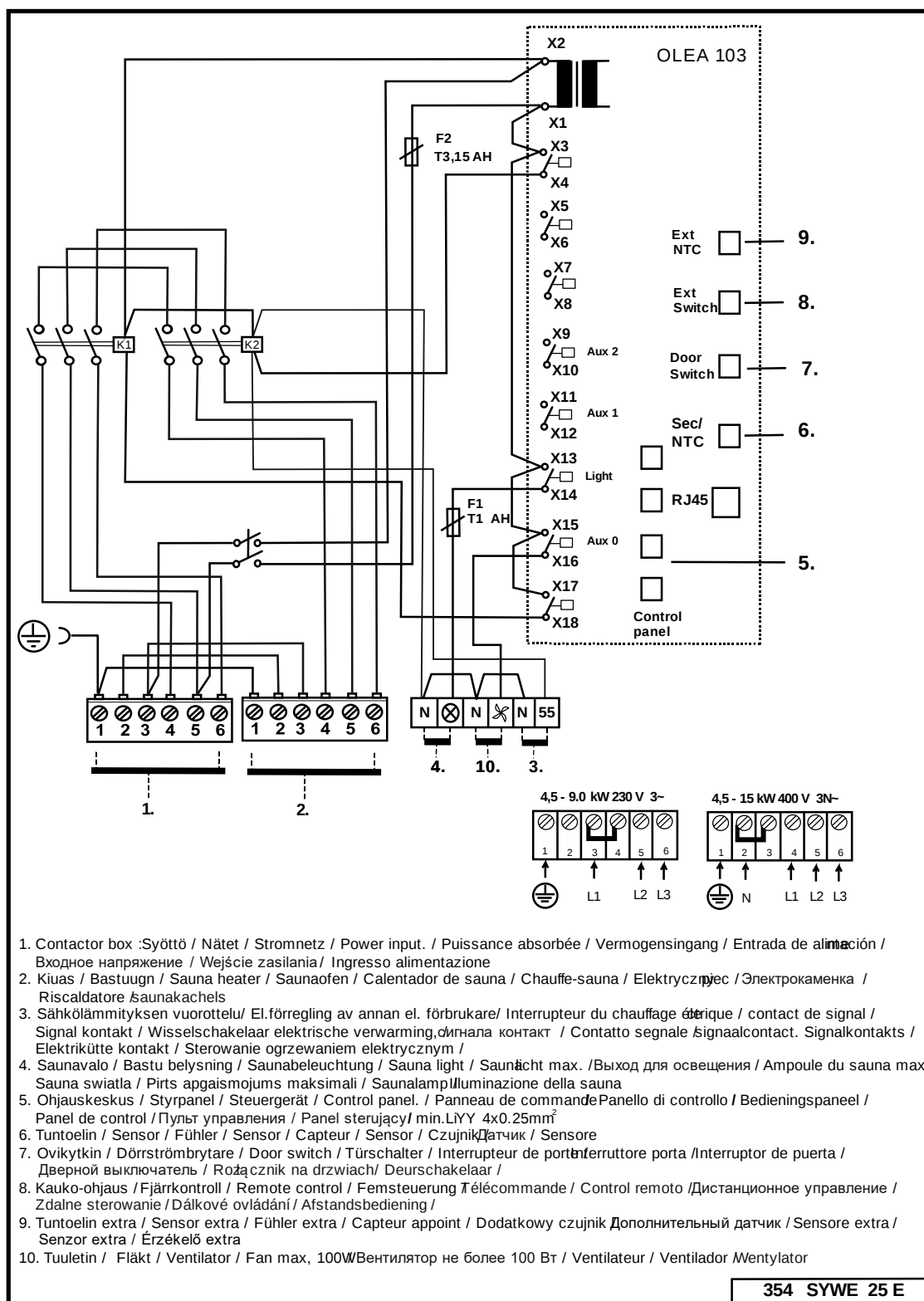
Figura 4 Diagrama de conmutadores WE 40
