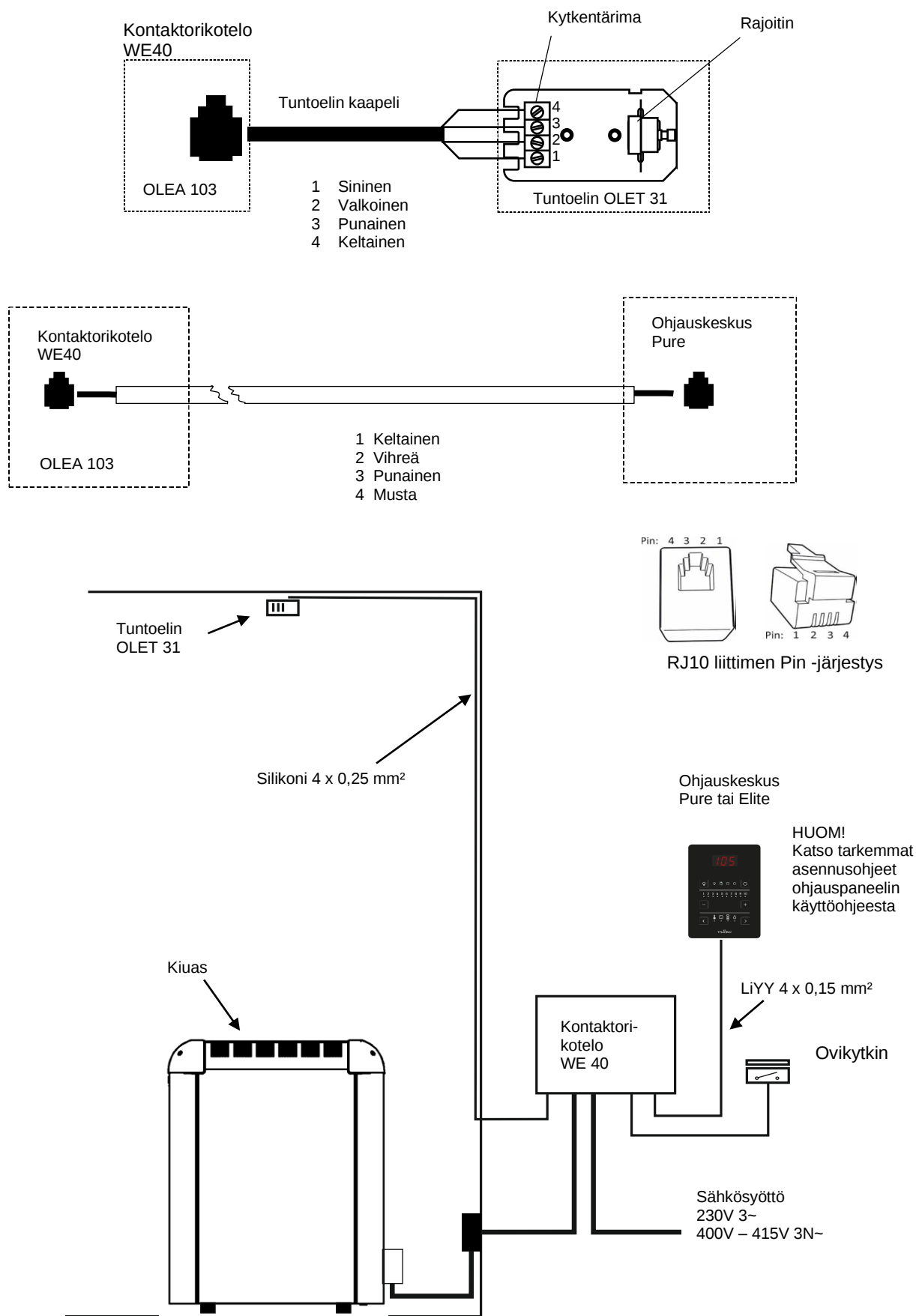
Kuva 5. Periaatekuva kytkennästä
