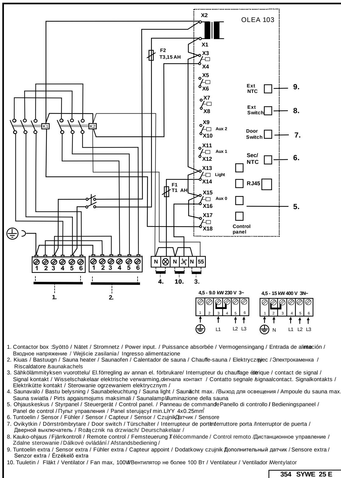
Bild 4 Kopplingsschema WE 40
