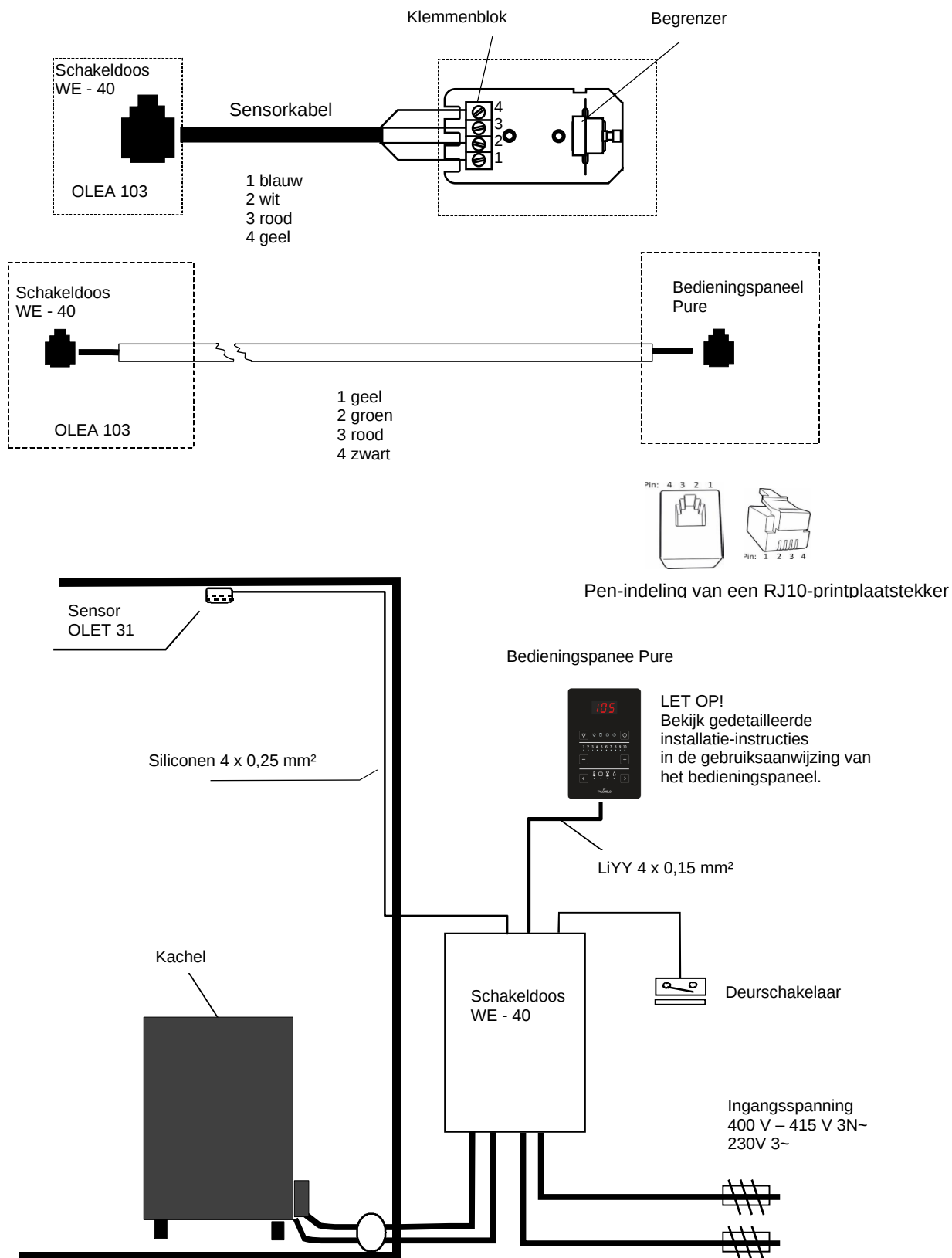
Afbeelding. 5 Principeschema van aansluitingen
