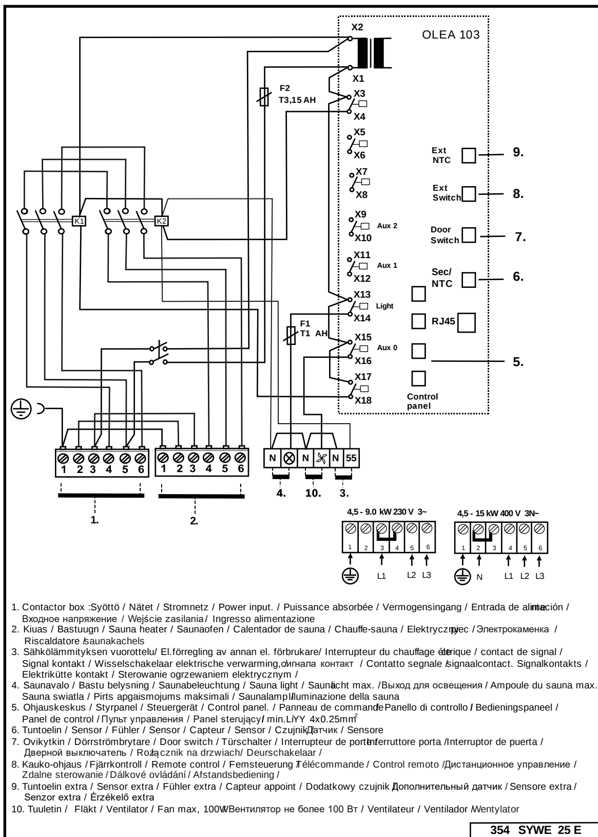
Abbildung 4 Schaltdiagram WE 40
